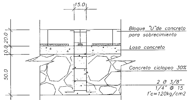
Detalle 4
