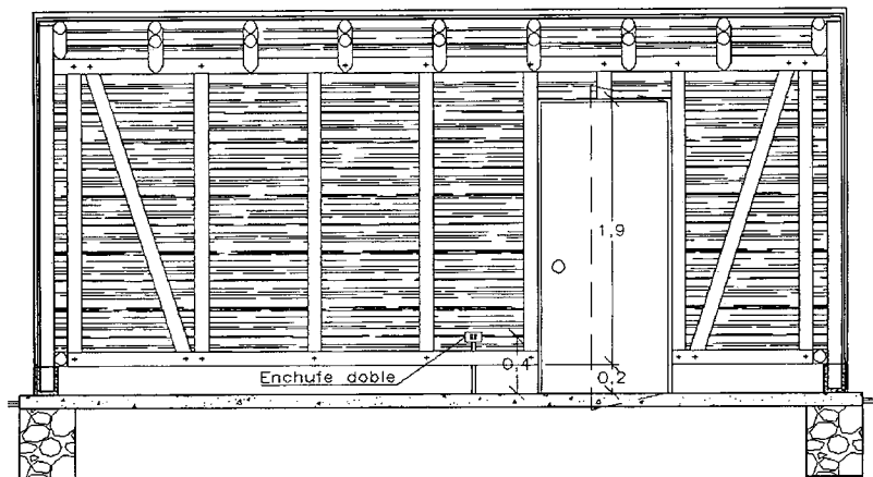
Corte 4-4
