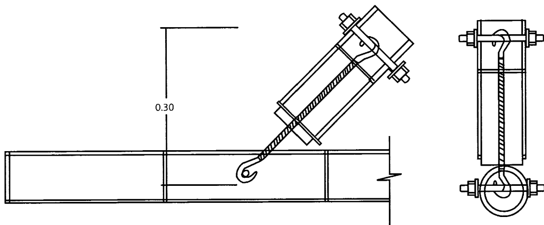
Corte
